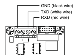
SA-232 wiring
